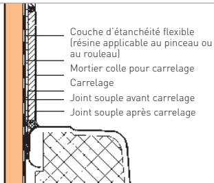
Figure 27 : Raccord horizontal d'une cloison simple peau avec un appareil receveur (douche, baignoire).
