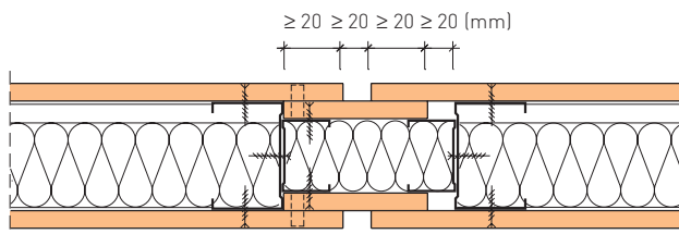
Coupe sur joint de dilatation – (montage de cloison FERMACELL à parement simple)
